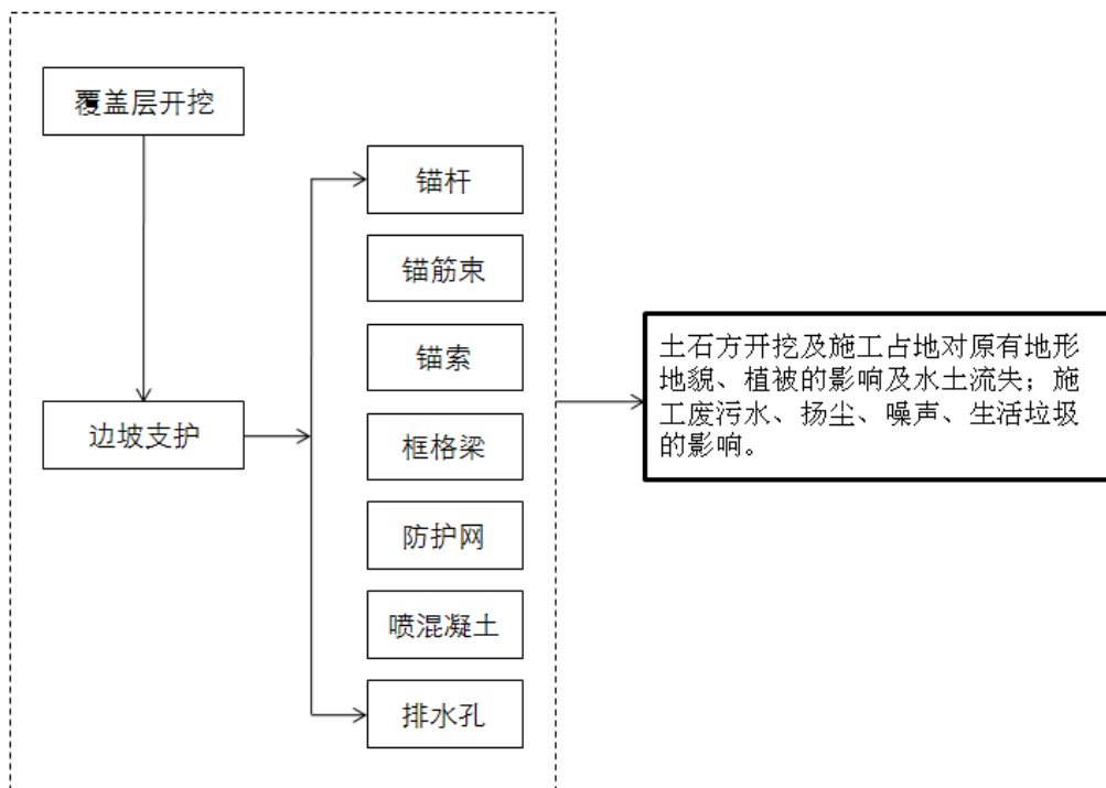
图4-2 边坡治理工程施工流程图
